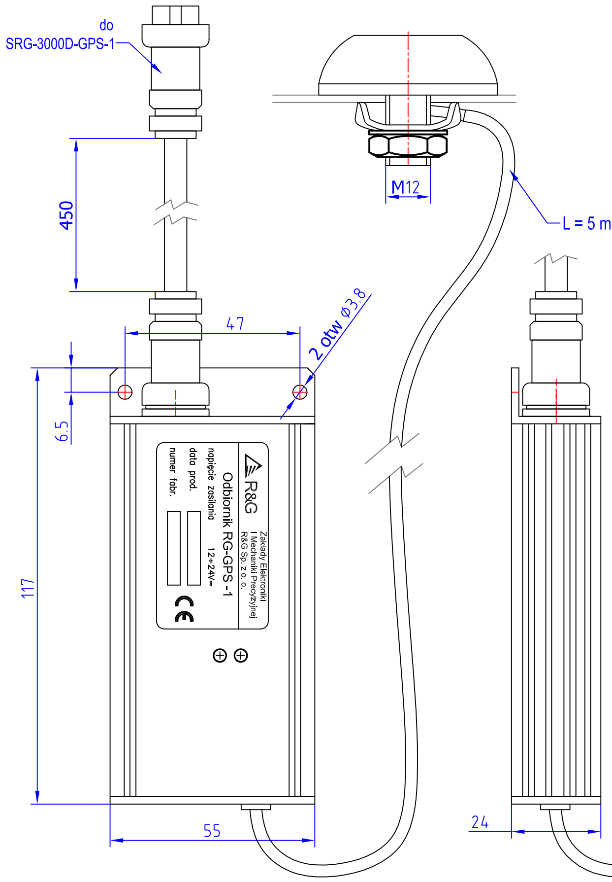
Wymiary gabarytowe odbiornika RG-GPS-1
