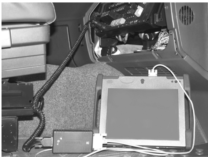
Abb. Diagnoseanschluss über Diagnostic Interface an den PC
