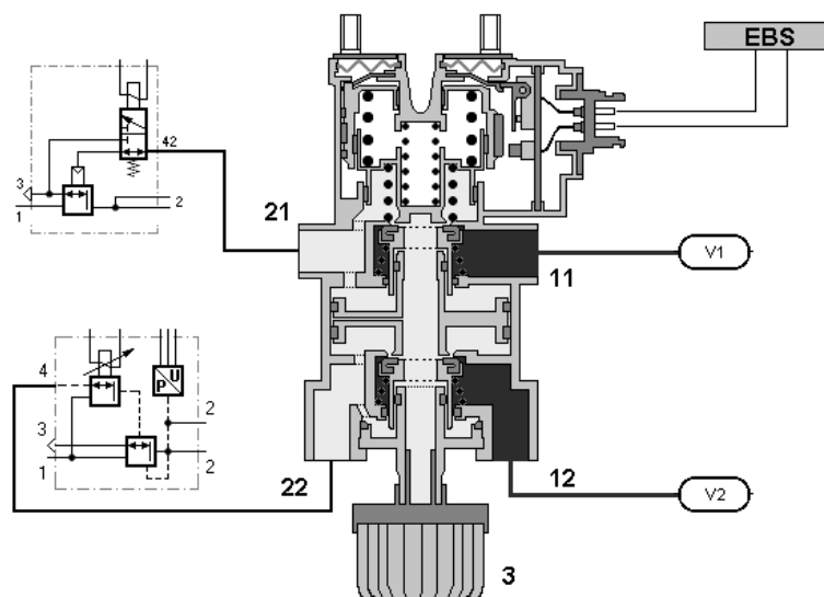
Abb. Funktionsweise des Bremswertgebers ohne Anschluss 4
