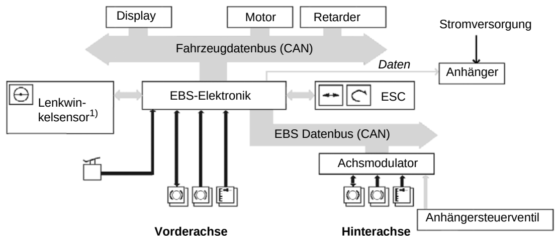
Abb. Anbindung von ESC an das Elektronische Bremssystem ab Variante 1C
